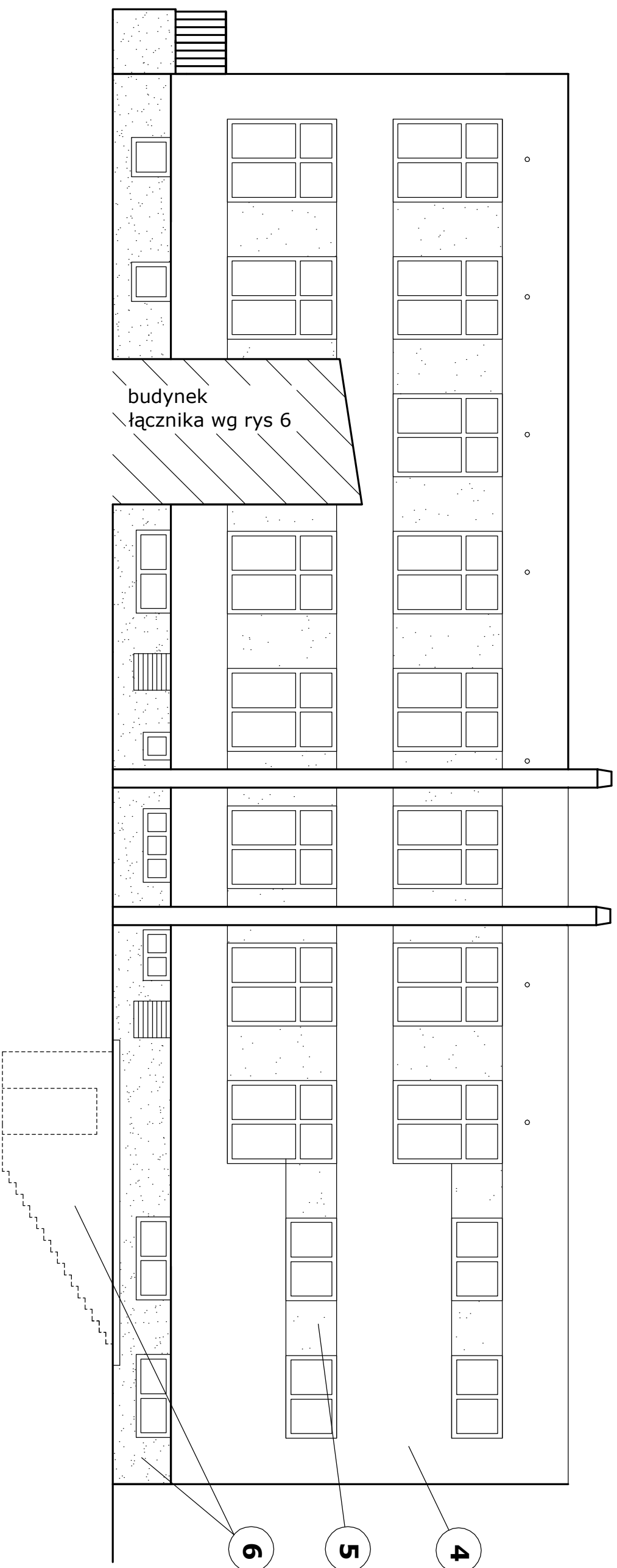
Elewacja południowa
