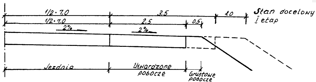
Rys. 3. Konstrukcja nawierzchni utwardzonego pobocza
