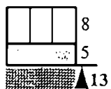
Rys. 4.3. Przekrój poprzeczny nawierzchni na wjeździe z betonowej kostki brukowej
