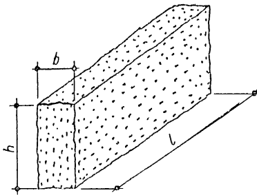
Wymiary krawężników
